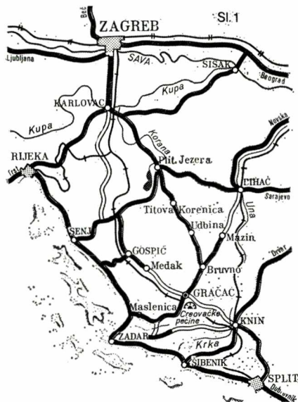
Sl. 1 Komunikacijski prilazi pećinama. Sl. 2 Međusobni odnos Gornje i Donje Cerovačke pećine. A—Ulaz u Gornju pećinu; B—Ulaz u Donju pećinu. 1—Lukačeva jama, 2—Dolinica ponor, 3—Nižanica ponor, 4—Mlinšte ponor, 5—Munžabin ponor, 6—Kesića ponor, (Projekcija njihovih odnosa nacrtana na topografsku osnovu)
