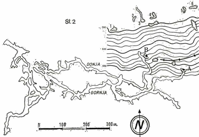
Sl. 1 Komunikacijski prilazi pećinama. Sl. 2 Međusobni odnos Gornje i Donje Cerovačke pećine. A—Ulaz u Gornju pećinu; B—Ulaz u Donju pećinu. 1—Lukačeva jama, 2—Dolinica ponor, 3—Nižanica ponor, 4—Mlinšte ponor, 5—Munžabin ponor, 6—Kesića ponor, (Projekcija njihovih odnosa nacrtana na topografsku osnovu)
